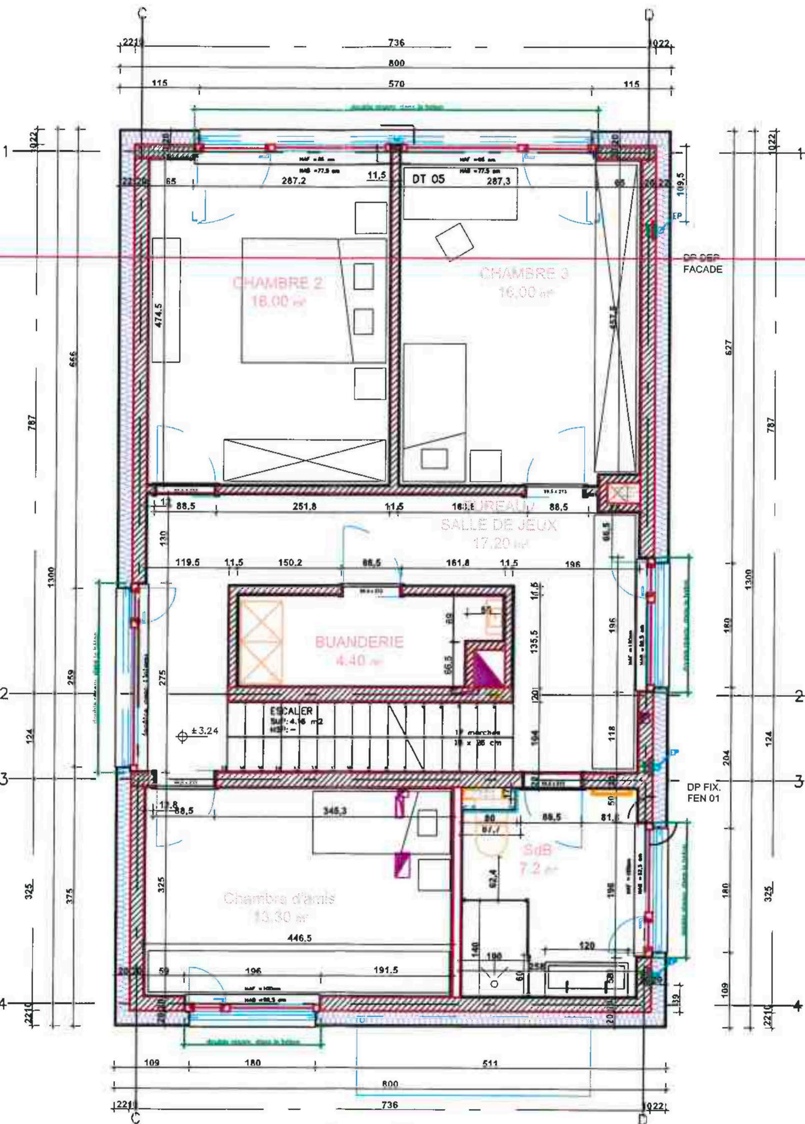
ÉTAGE +1 ECH 1:50
