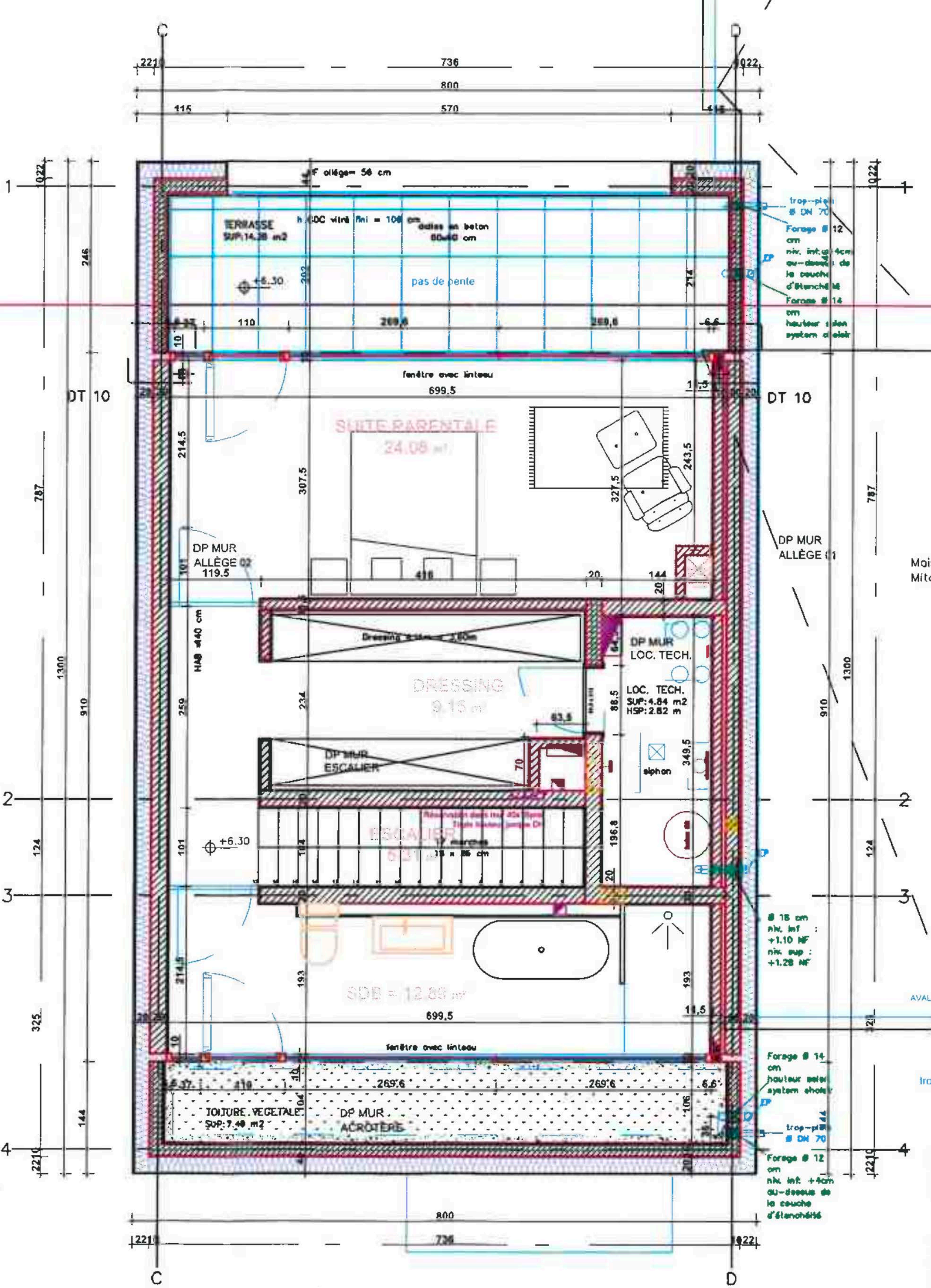
ÉTAGE +2, COUPE ALLÈGE BAS ECH 1:50
