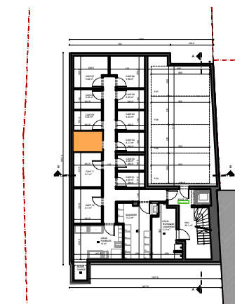
SOUS-SOL -02 (CAVES)
