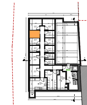
SOUS-SOL -02 (CAVES)
