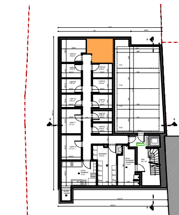
SOUS-SOL -02 (CAVES)
