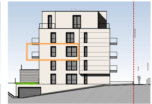
FACADE LATERALE GAUCHE
