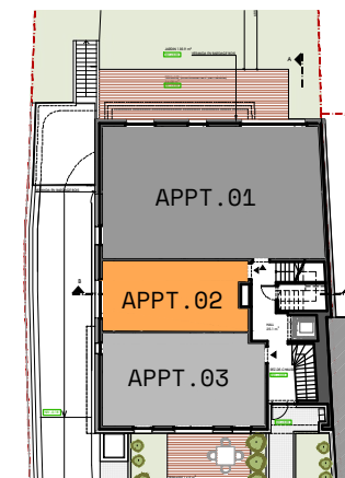
REZ-DE-CHAUSSEE
