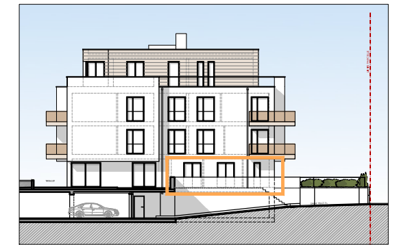
FACADE LATERALE GAUCHE
