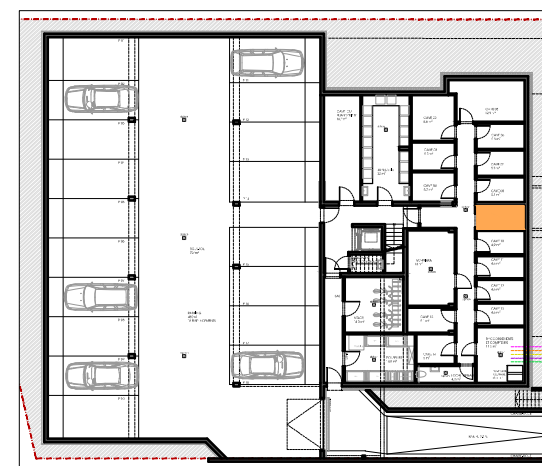
SOUS-SOL -01 (CAVES)
