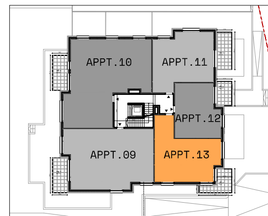
ETAGE +02
