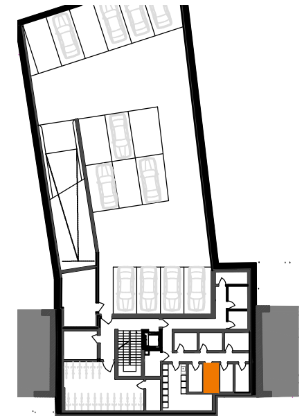
SOUS-SOL -1 (CAVES)
