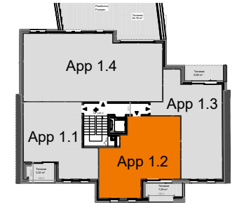
ETAGE +1
